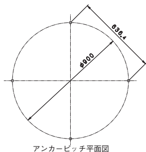
アンカーピッチ平面図
