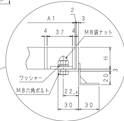
ボルト固定部分拡大図
