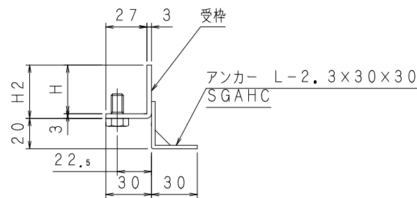
ボルト固定部分拡大図
