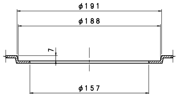
流し台金具取付部絞り寸法
