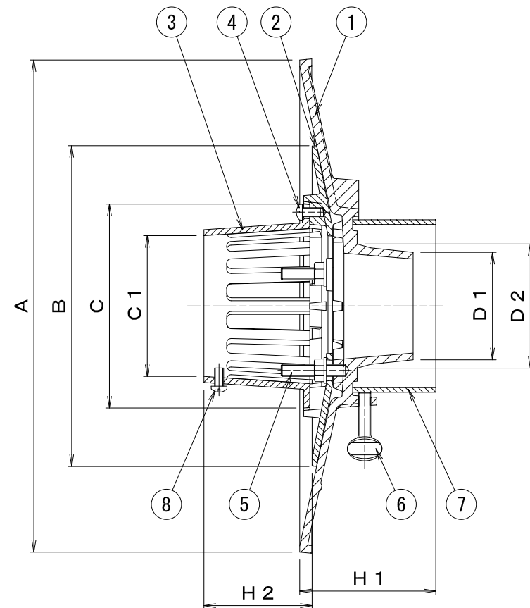
■寸法表 (SV1BK)
